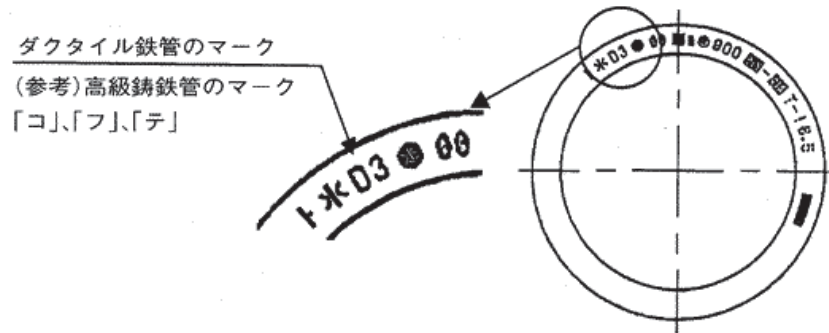
【高級鑄鉄管】
