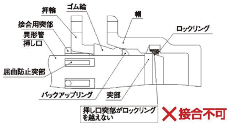
NS形異形管挿し口（呼び径75～250）と帽の接合
